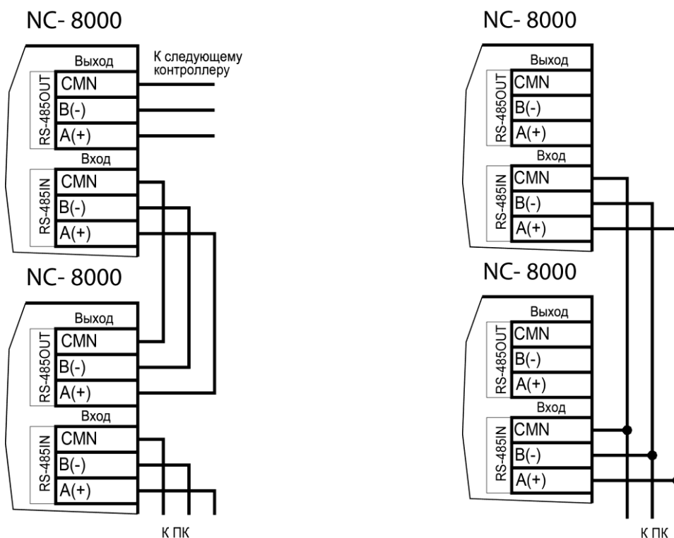
Рисунок 26. Схема соединения контроллеров по топологии «Шина» Рисунок 27. Пример соединения контроллеров по топологии «Звезда»
